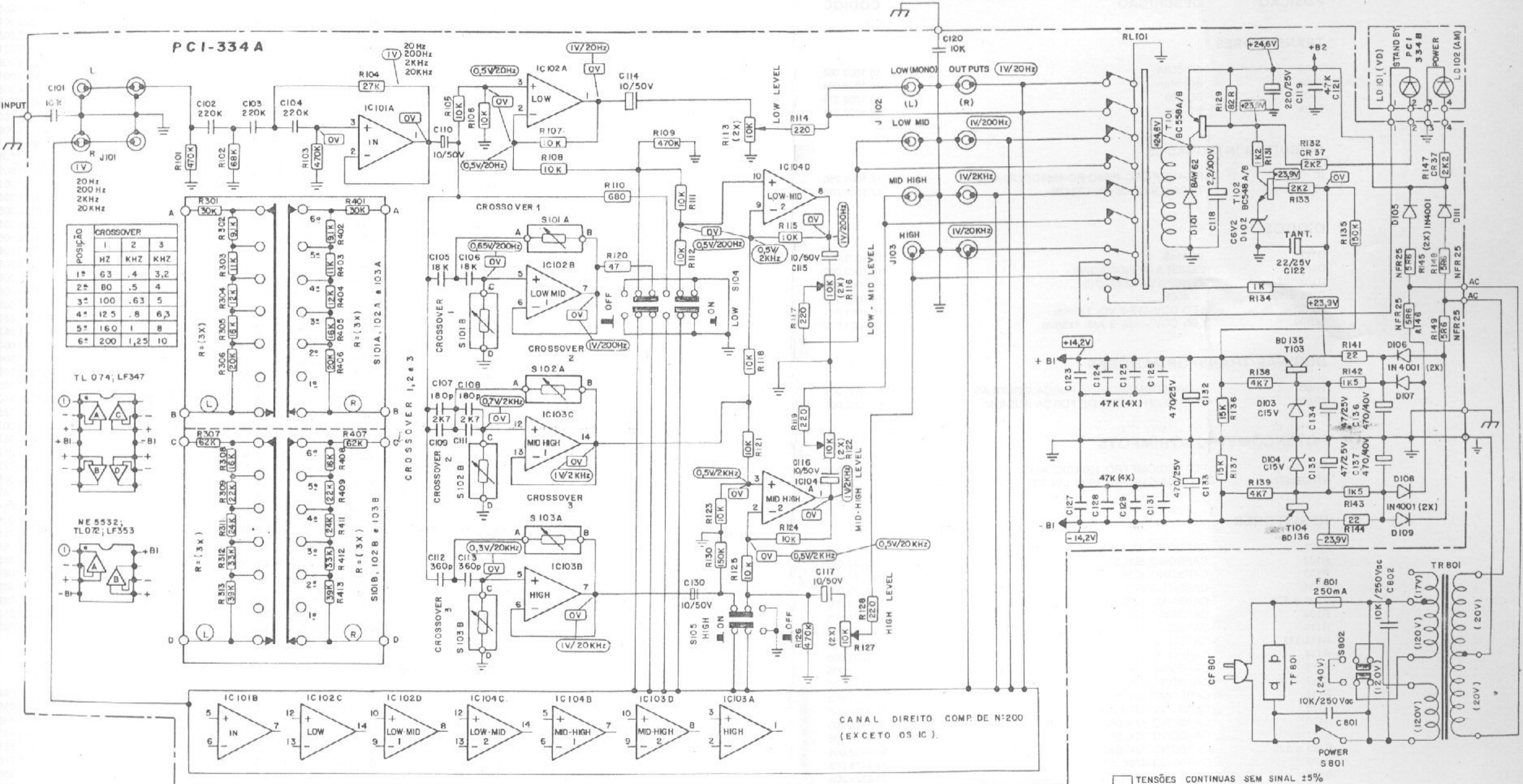
Diagrama Elétrico - CX-II - Stereo Electronic Crossover Gradiente
